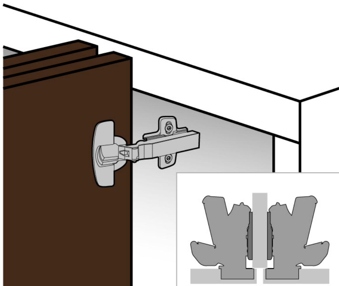
Montage en demi-applique
