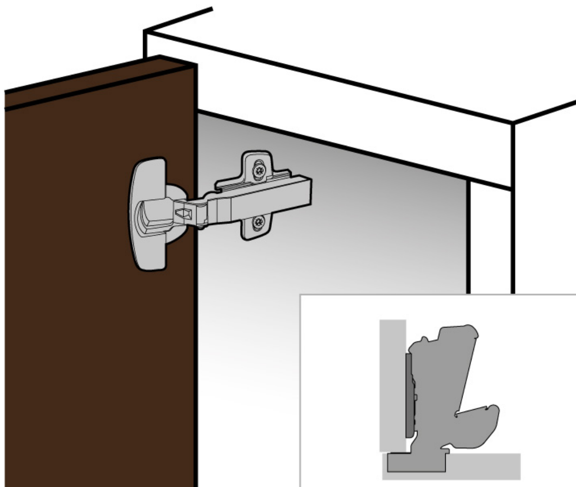
Montage en applique
