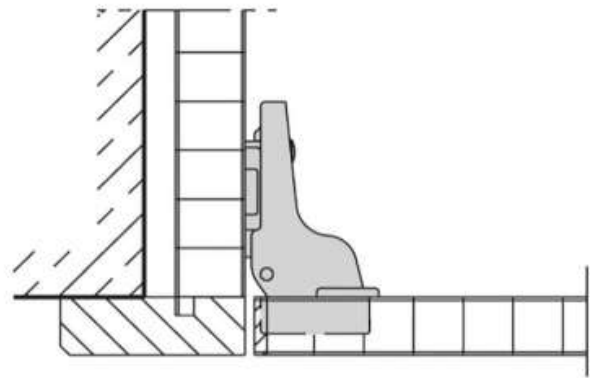
vantail intérieur
