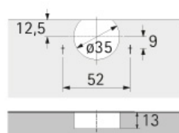
Cotes de perçage TX32/52x9 Selekt Pro 2000
