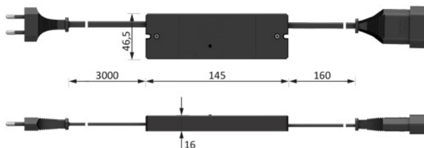
31.110.01 Smartempfänger smartreceiver 230/240VAC (keine Dimmfunktion no dimming)
