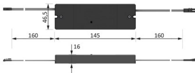
31.110.01 Smartempfänger smartreceiver 230/240VAC (keine Dimmfunktion no dimming)
